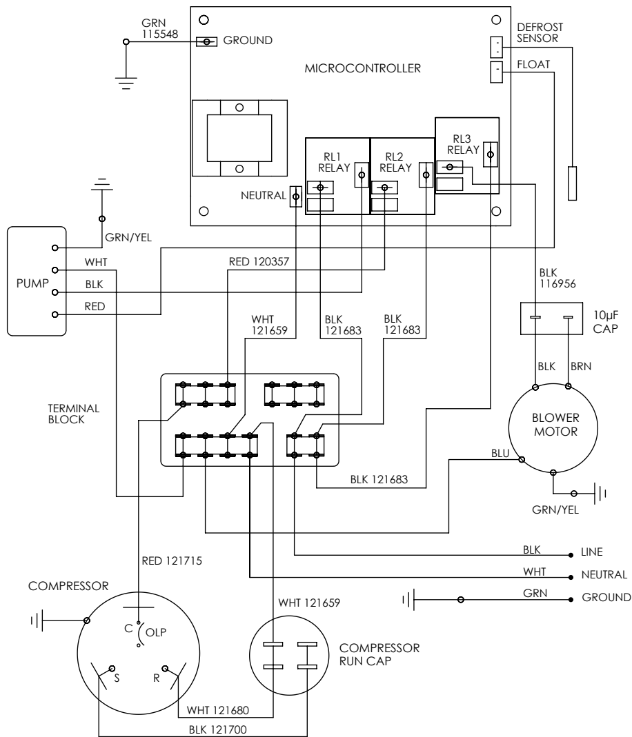
WIRING SCHEMATIC
