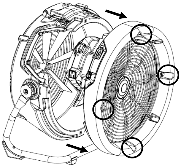
Fig. C: Apilado para almacenami-ento o transporte
