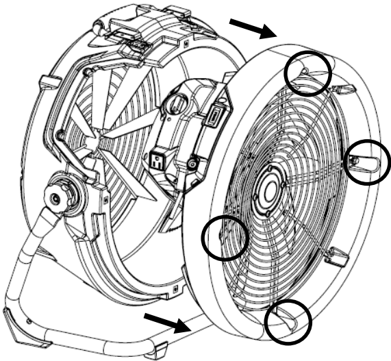
Fig. C: Superposition pour le stockage ou le transport
