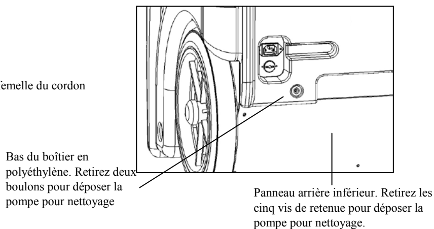
FIG. D : PANNEAU D'ACCÈS DE LA POMPE
